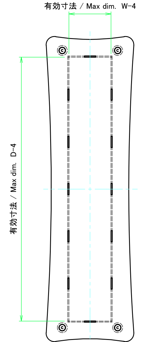
下カバー / Bottom cover
