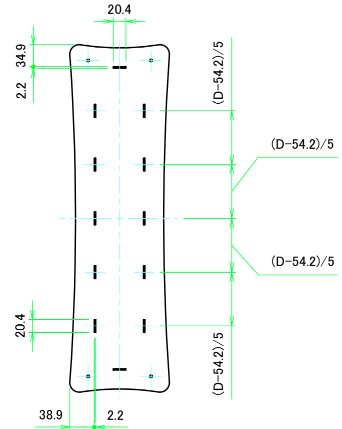
上カバー裏面 / Top cover Backside
