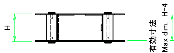
Wパネル1 / W panel 1
